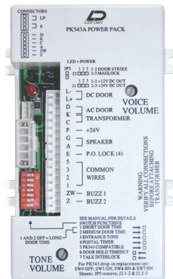
PK-543A POWER PACK
